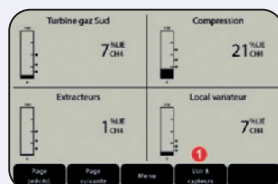
Affichage simultané 4 capteurs
